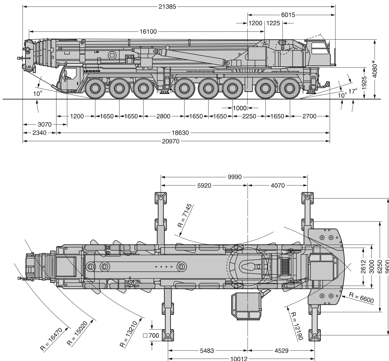
外観寸法
