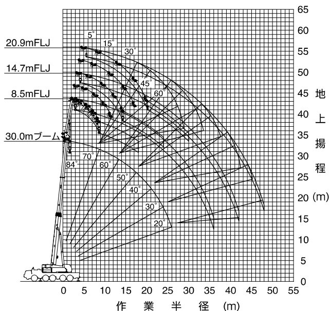
30.0mブーム+1.85m+フルオートラフinggジブ
