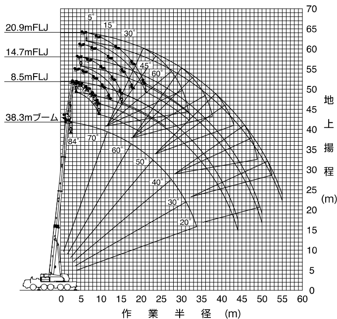
38.3mブーム+1.85m+フルオートラフinggジブ
