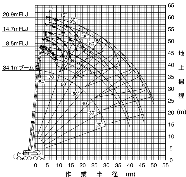
34.1mブーム+1.85m+フルオートラフinggジブ
